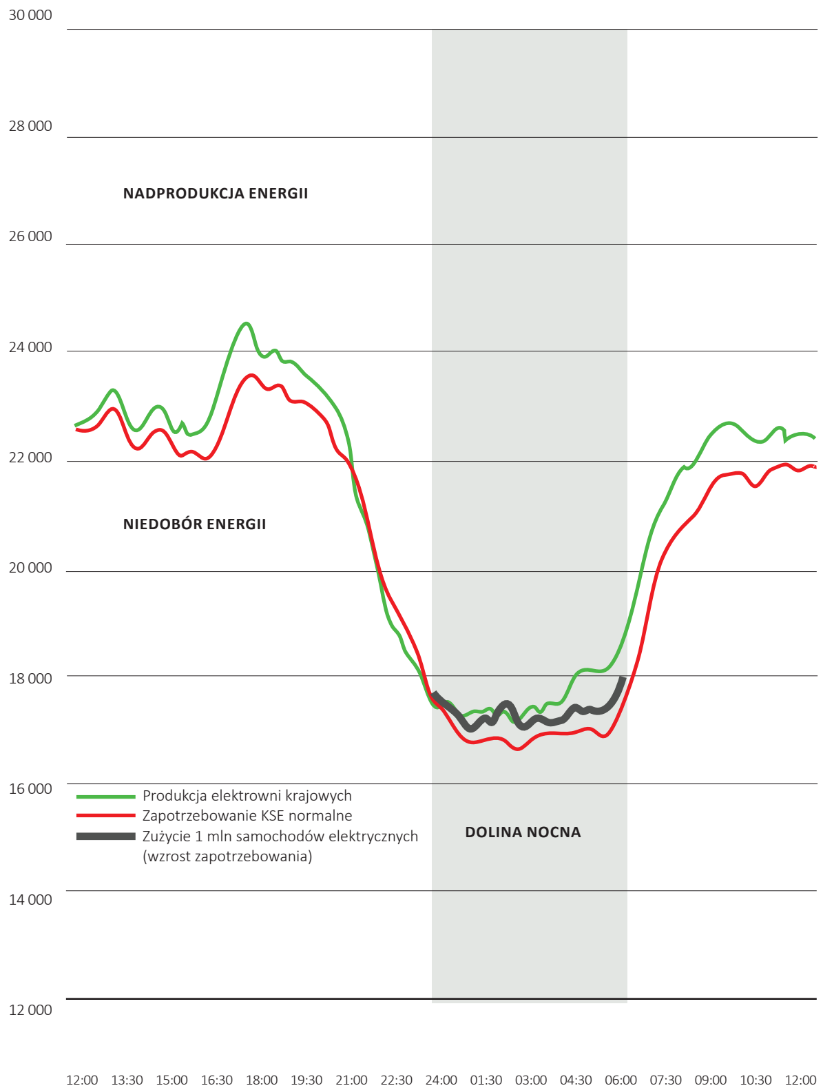
RYS. 1 ZAPOTRZEBOWANIE KSE I PRODUKCJA ELEKTROWNI KRAJOWYCH [MW]
